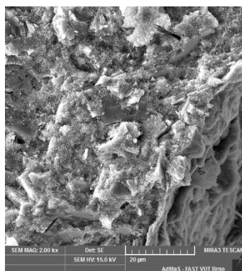
Foto 1: Beton bez příměsi POROSTOP IN Foto 2: Beton s příměsí POROSTOP IN
